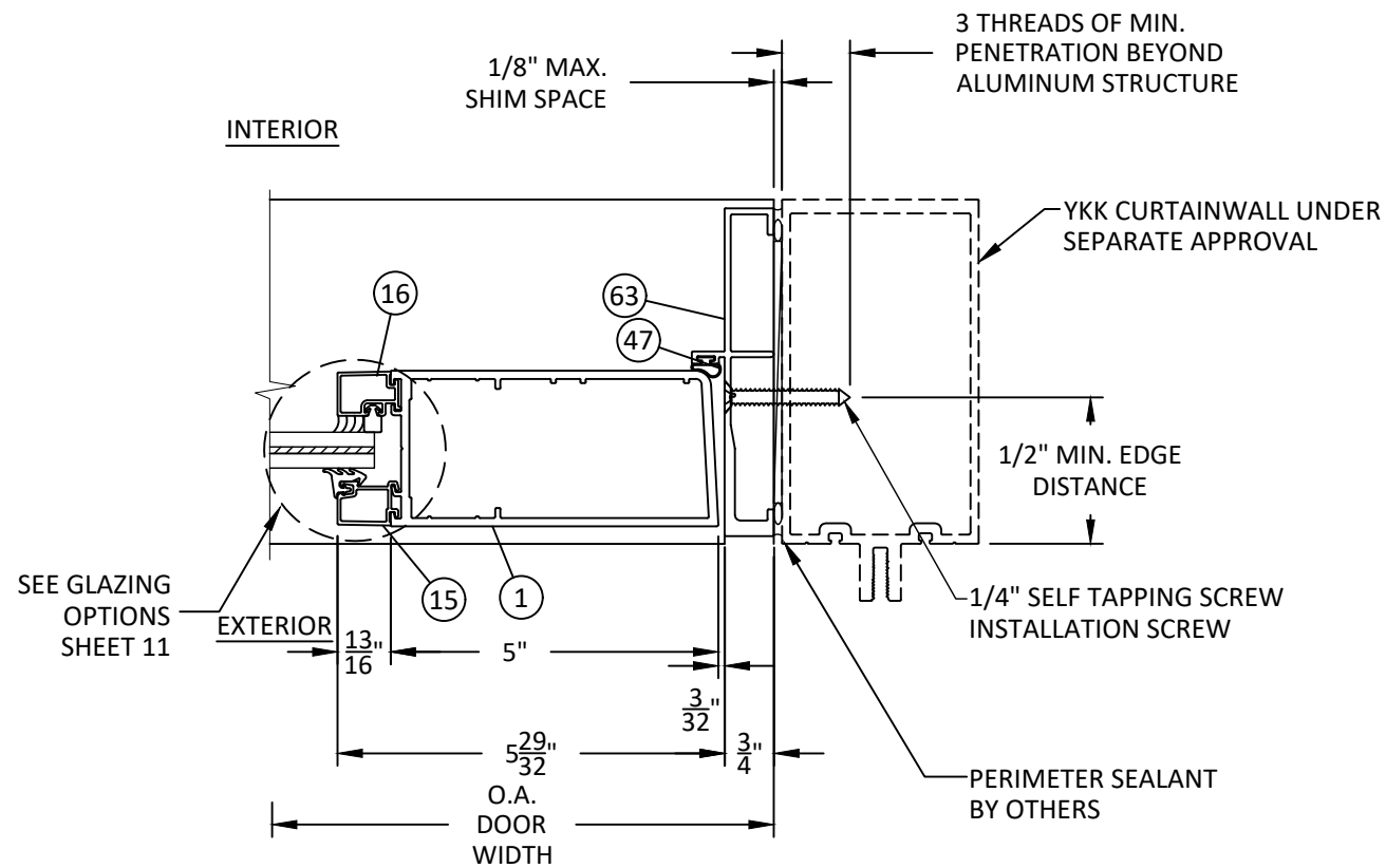
N9 HORIZONTAL SECTION JAMB - TYP. CURTAINWALL MULLION
