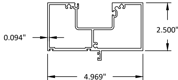
73 I.G. TRANSOM MULL 6063-T5
