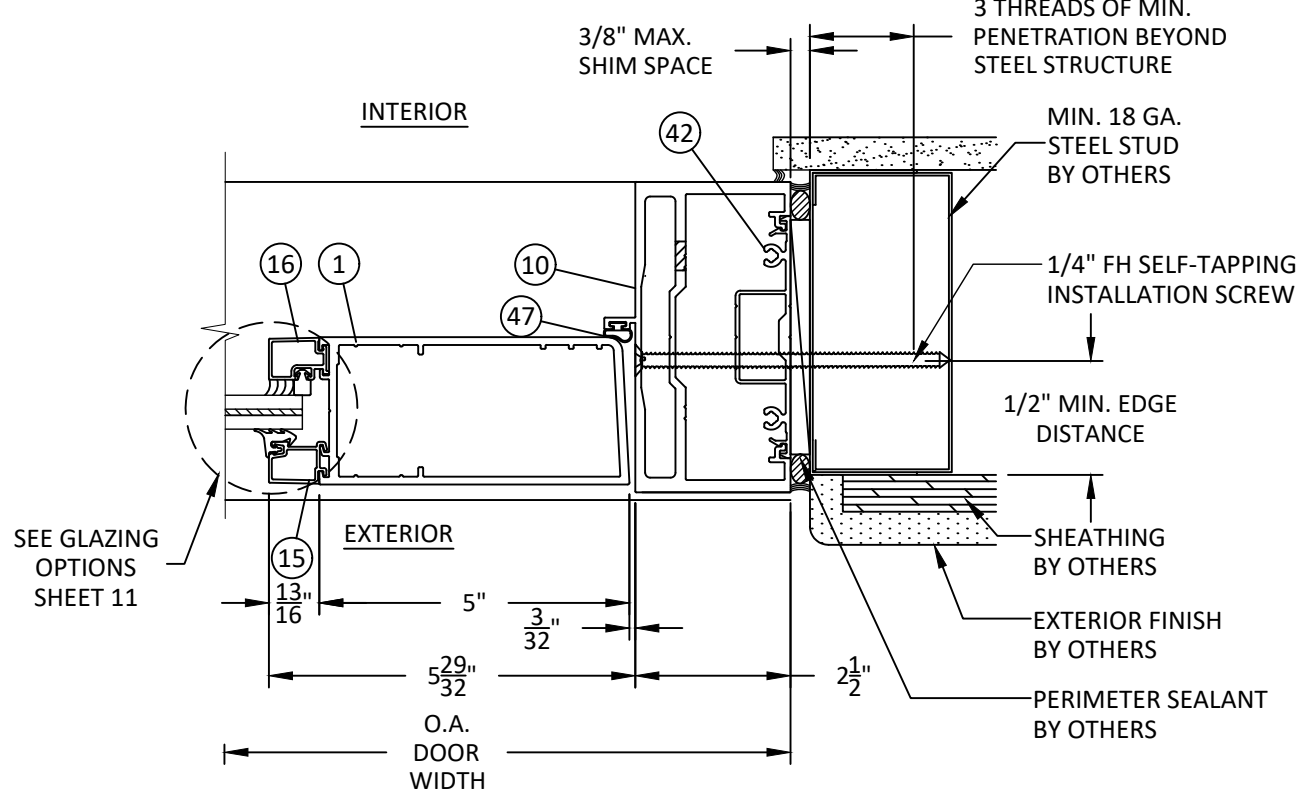
J HORIZONTAL SECTION 8 JAMB - STEEL STUD
